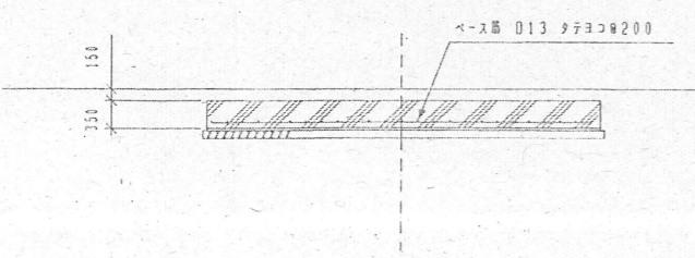
F1 断面 S=1:50
