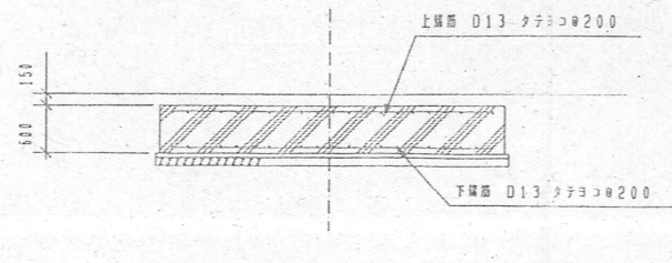
F2-F4 断面 S=1:50
