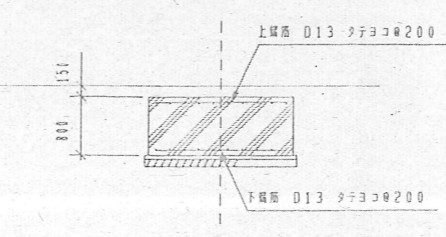
F5 断面 S=1:50
