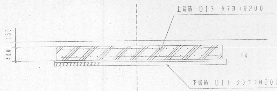
F4 基礎図 S=1:50
