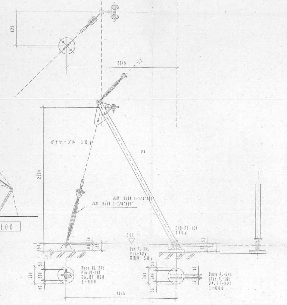
P4まわり詳細図 S=1:20
