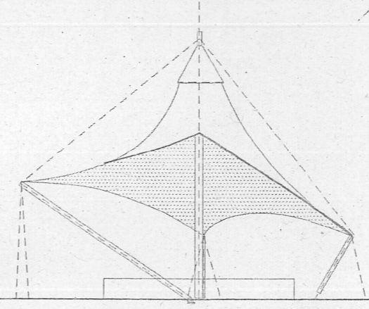
断面図 S=1:100
