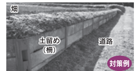
法面に土留め(柵)を設置
