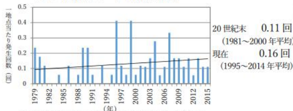
図 千葉県内17地点において時間降水量50mm以上となった回数(1地点当たり)の経年変化 直線は2次回帰による近似直線。回数は1地点当たりの平均。 (気象庁HPのアメダスデータをもとに作成)
