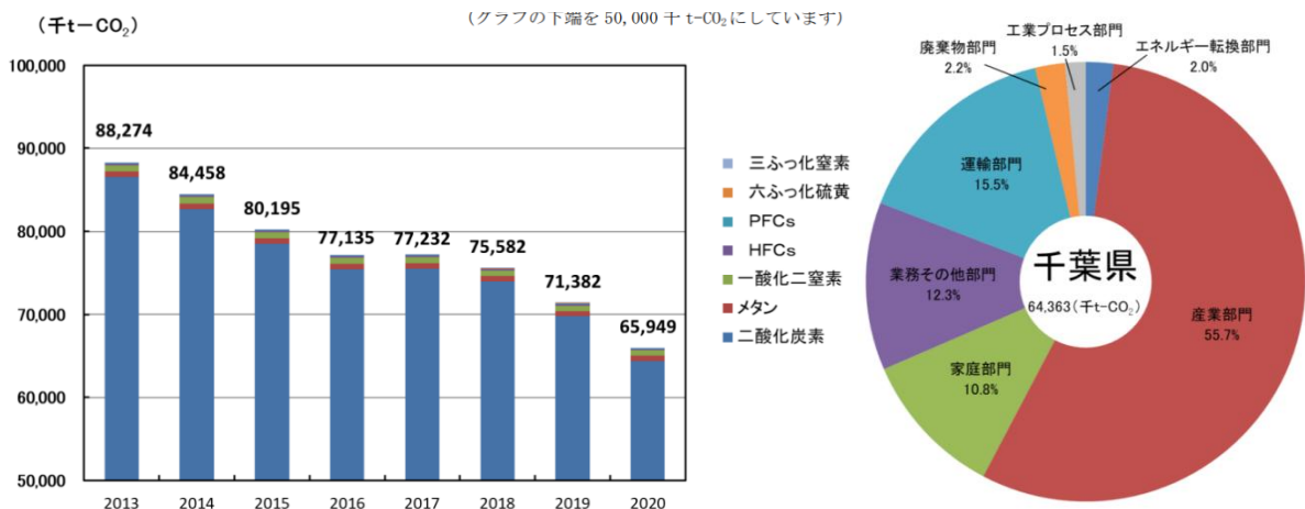
図 3.3 千葉県の温室効果ガス排出量
