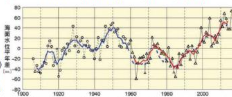
図 日本沿岸の年平均海面水位の経年変化 1906～1959年が日本4地点(北海道忍路、石川県輪島、島根県浜田、宮城県細島)、1960年以降は16地点の観測所の観測値。青色の実線は4地点の5年移動平均値、1960年以降の青色破線も同4地点の5年移動平均値である。平成23年(2011年)東北地方太平洋沖地震の影響を受けた4地点(函館、深浦、柏崎、八戸)は2011年以降のデータを使用していない。 気象庁HP「海洋の健康診断表:日本沿岸の海面水位の長期変化傾向」(H29.3)から
